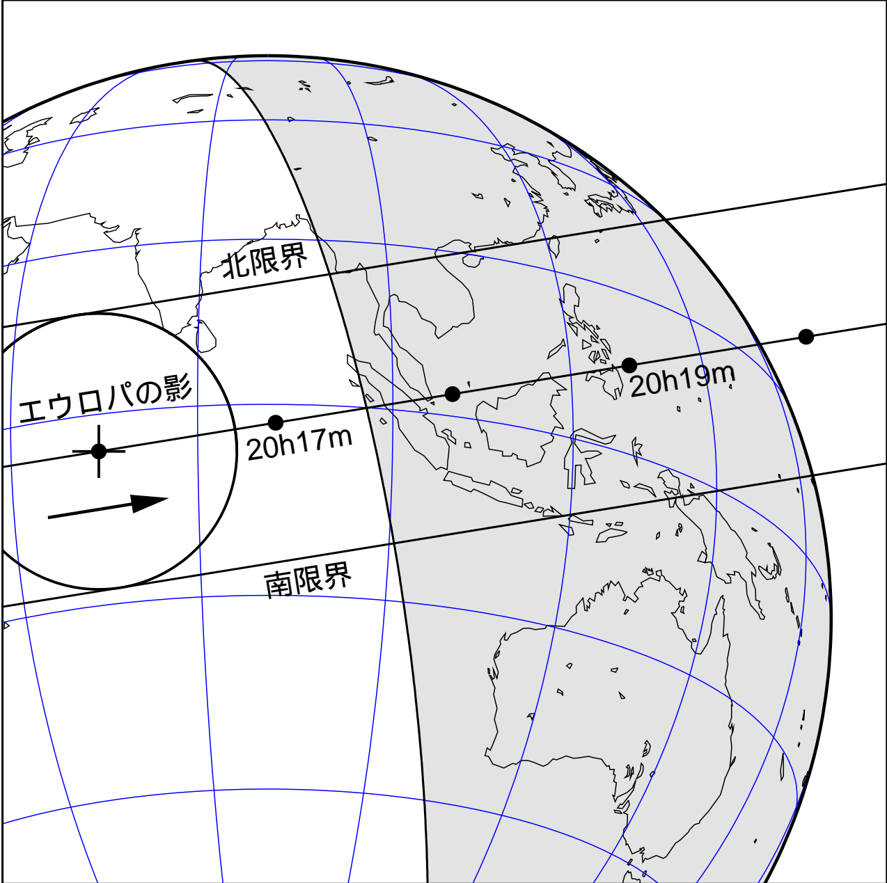
エウロパの掩蔽帯(JST)
