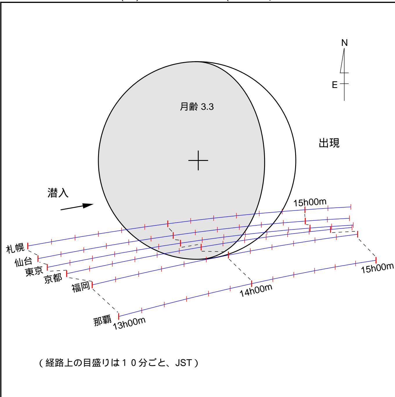
図1 2021年11月8日(月) 昼間の金星食 (-4.6等)
