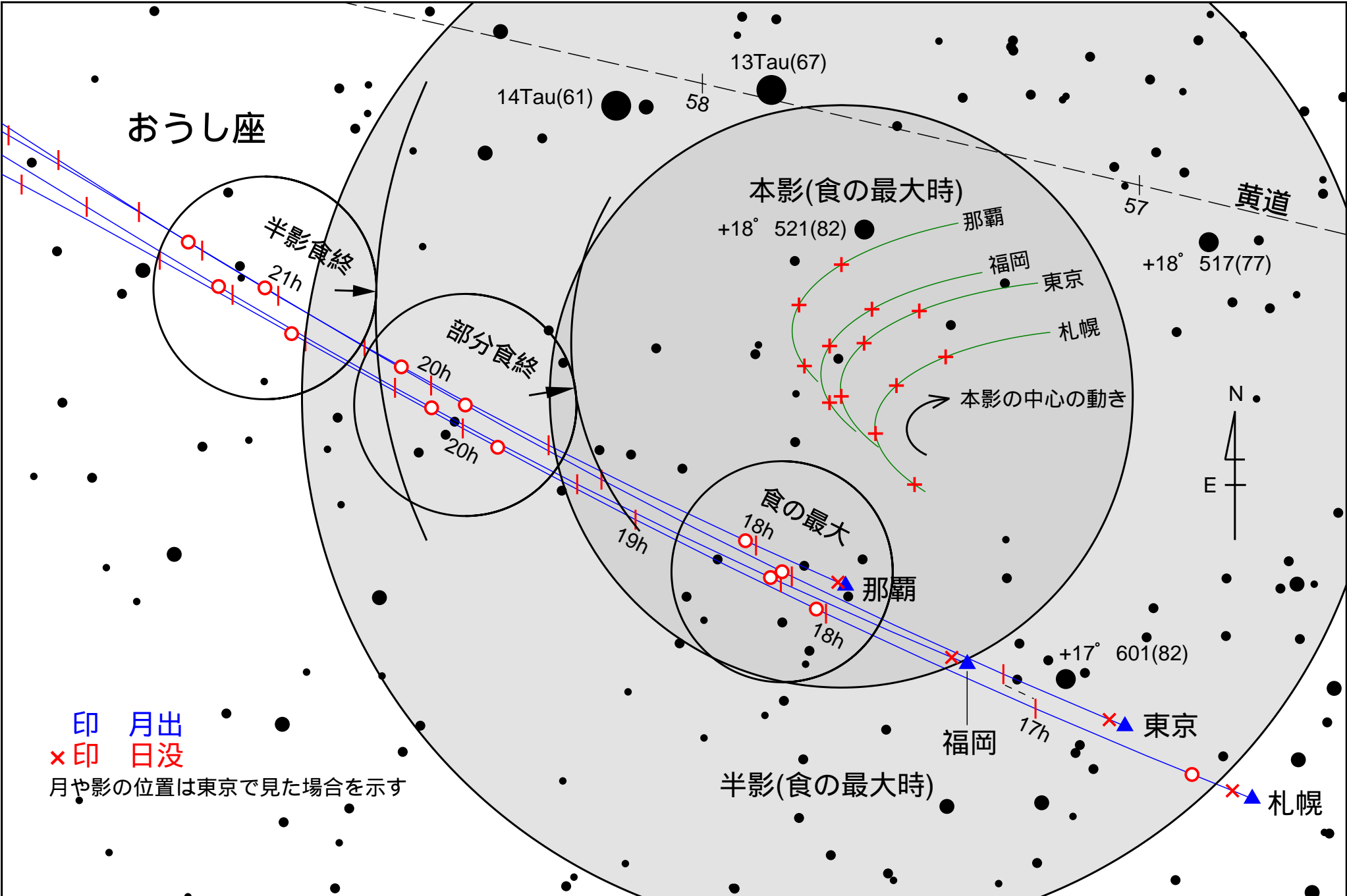
図5 食の最大時の星野(2021年11月19日(金))
