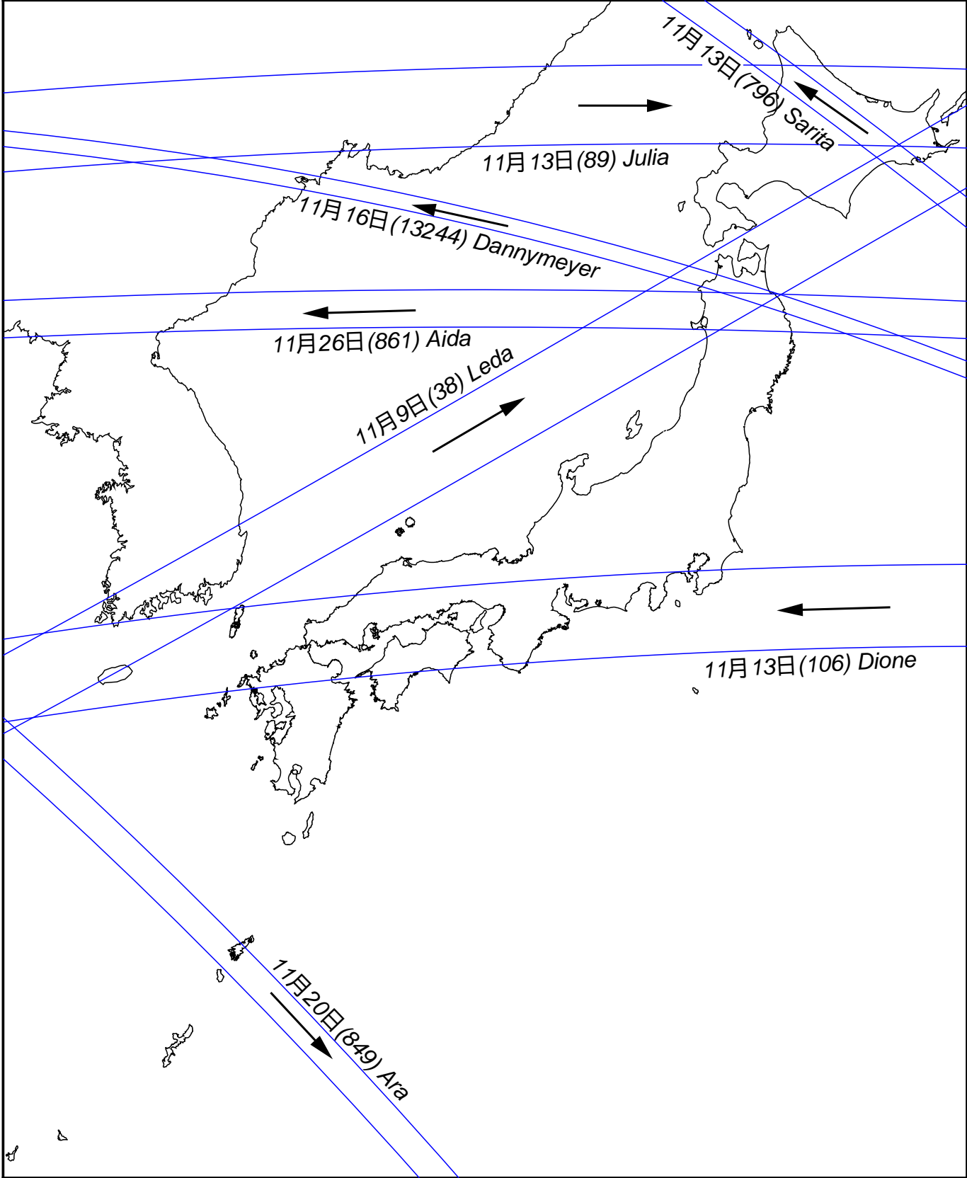
図9 小惑星による主な掩蔽帯経路 ( S.Preston予報ほか ) 2021年11月 矢印は影の移動方向を示す
