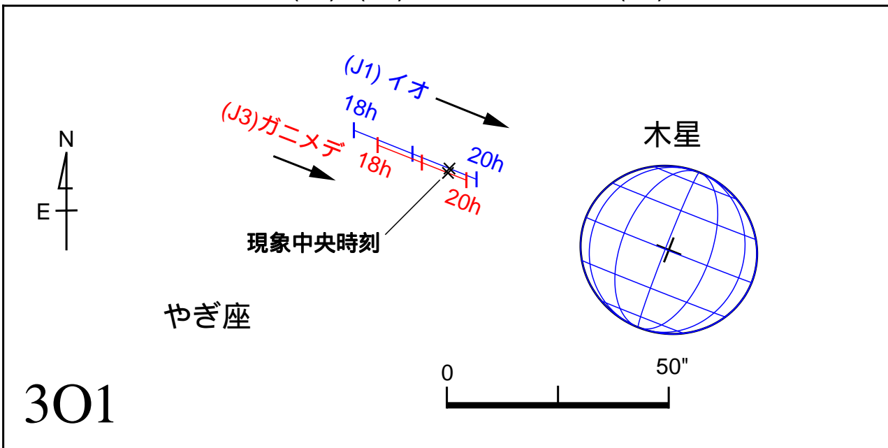
図6 2021年11月16日(火) (J3)ガニメデによる(J1)イオの掩蔽
