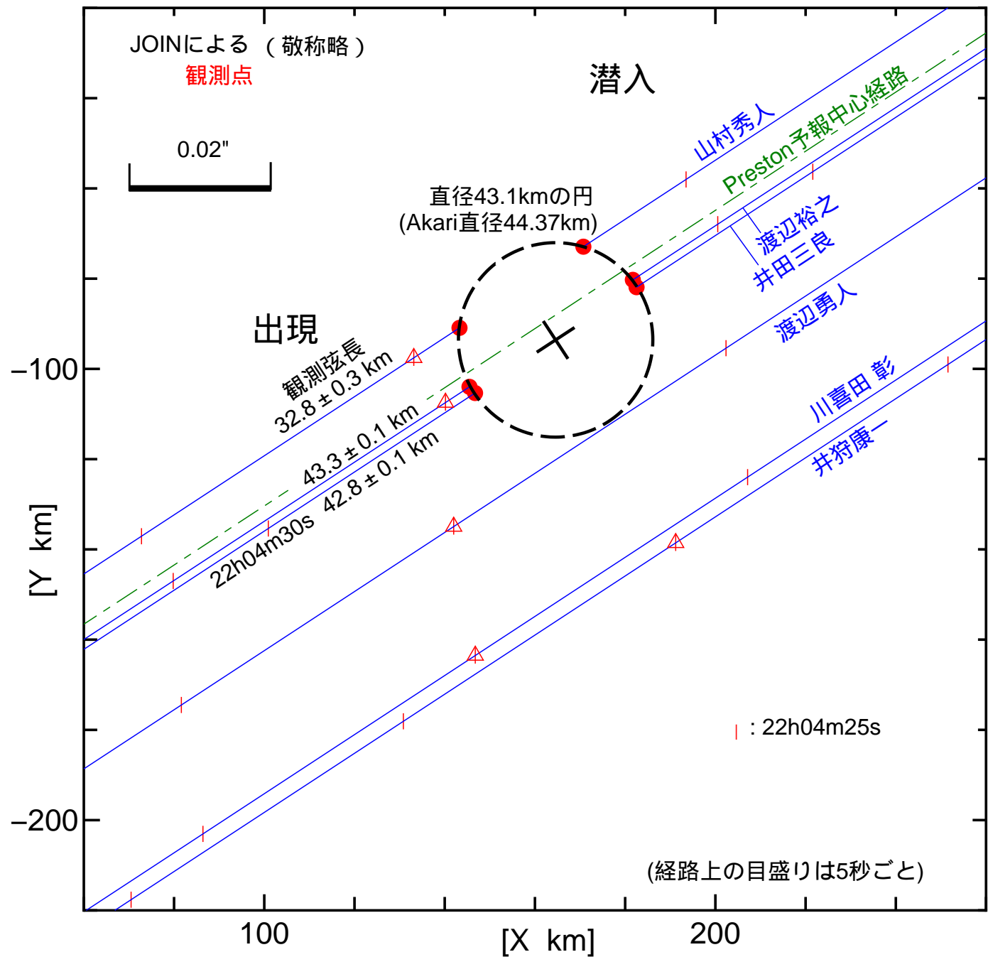
図8 (2326) Tololo (2021年4月5日) の食 観測結果 (時刻はJ.S.T)
