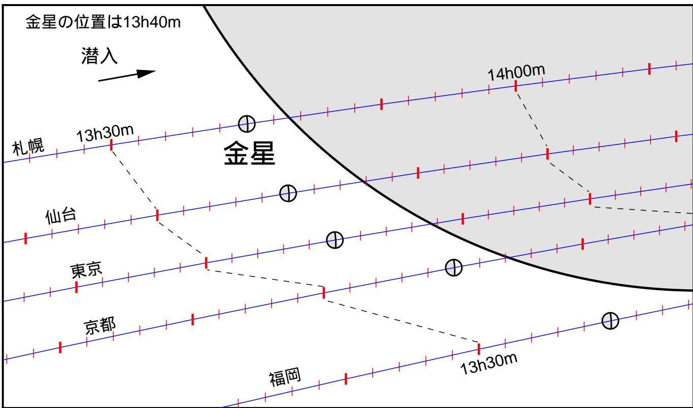
図2 金星の潜入・出現の様子
