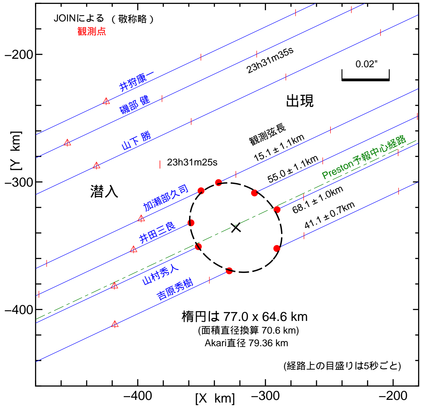
図7 (795) Fini (2021年3月10日) の食 観測結果
