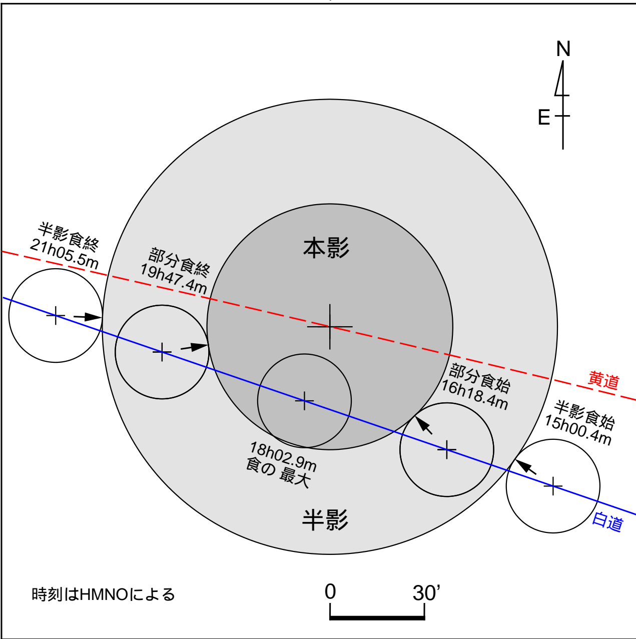
図4 2021年11月19日 部分月食(地心) JST
