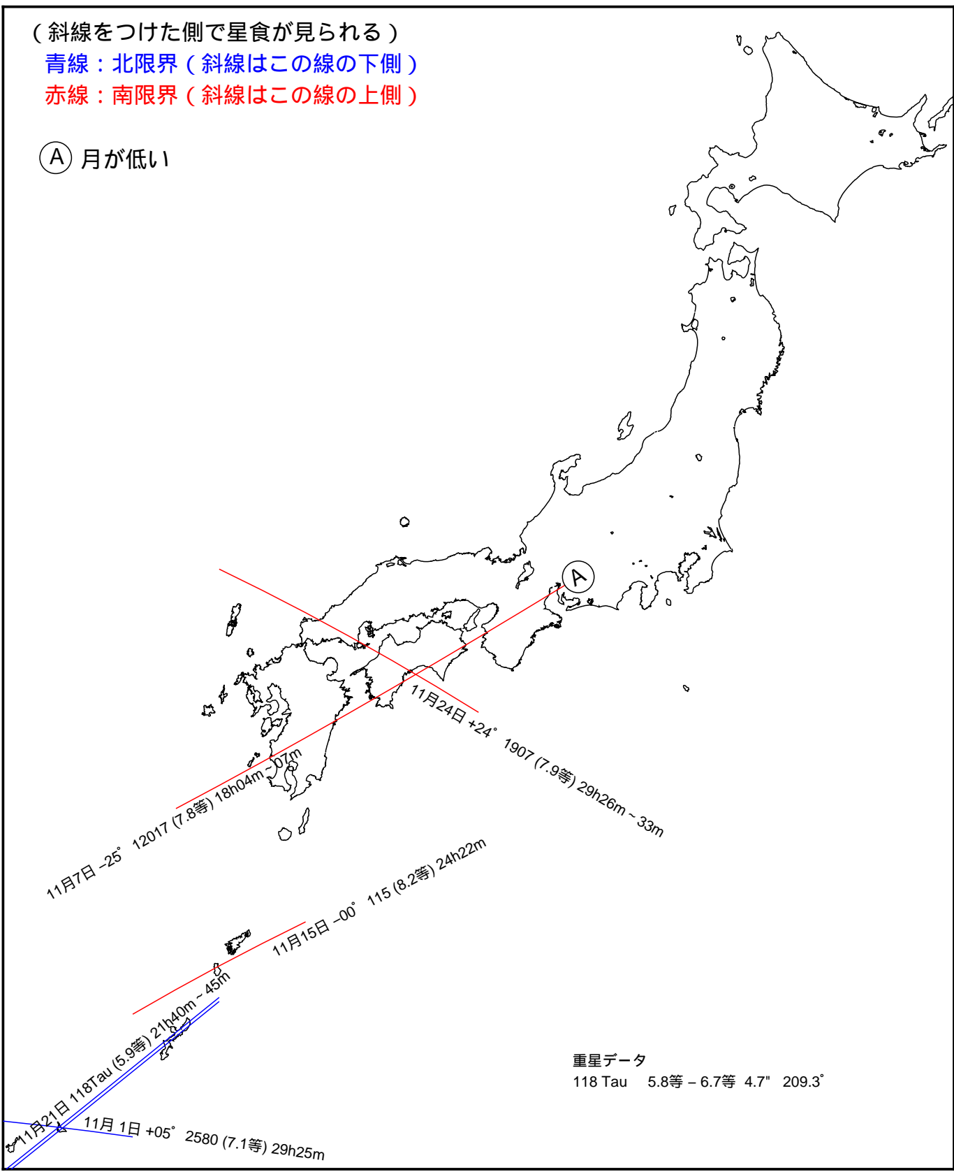
図10 2021年 11月 日本を通る主な星食限界線
