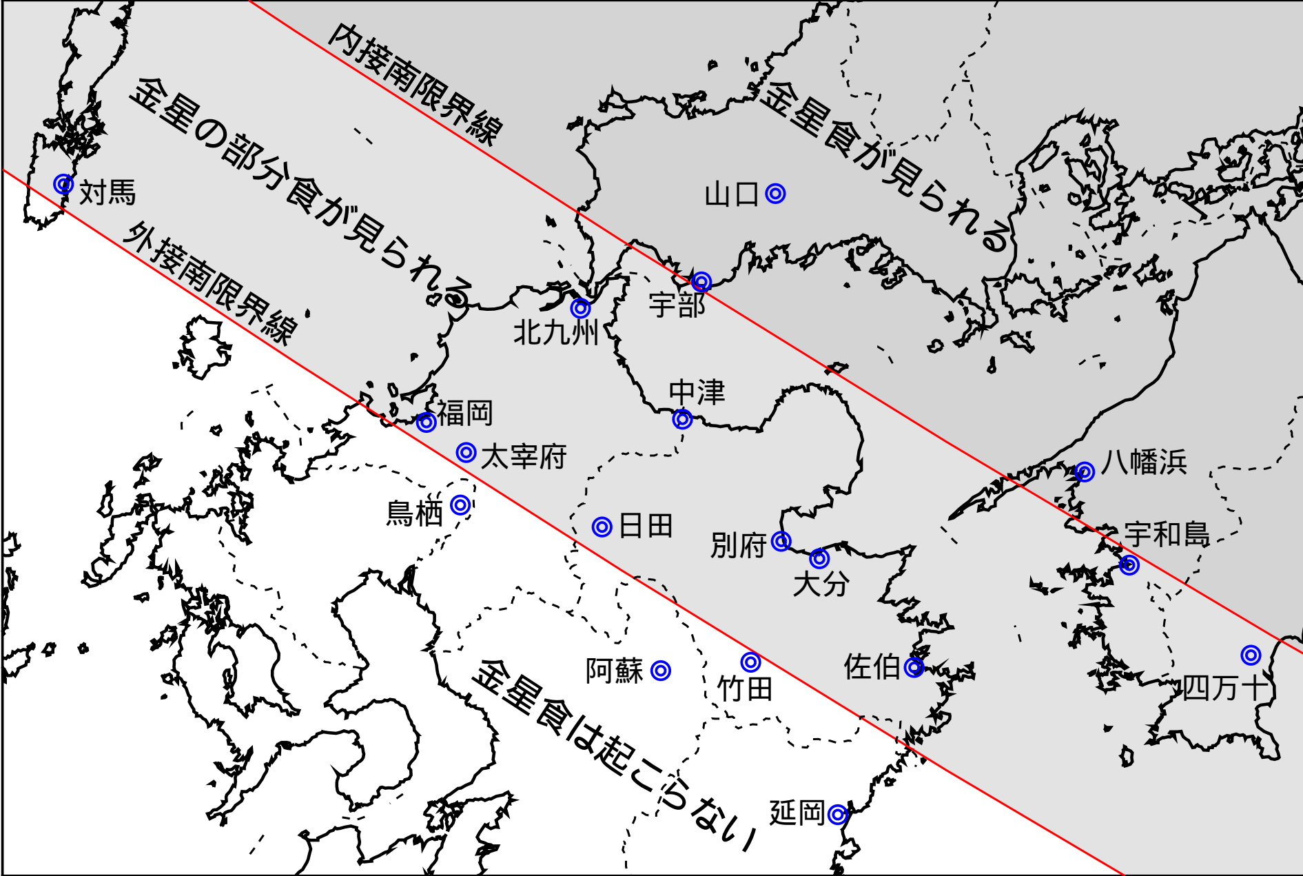
図3 金星食の南限界付近
