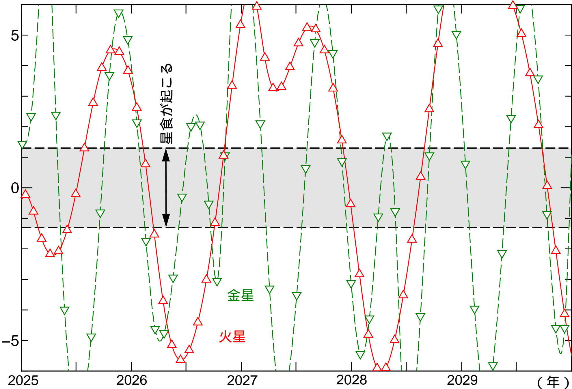
図3a 金星・火星食ダイヤグラム (目盛りは毎年1月1日と7月1日)
