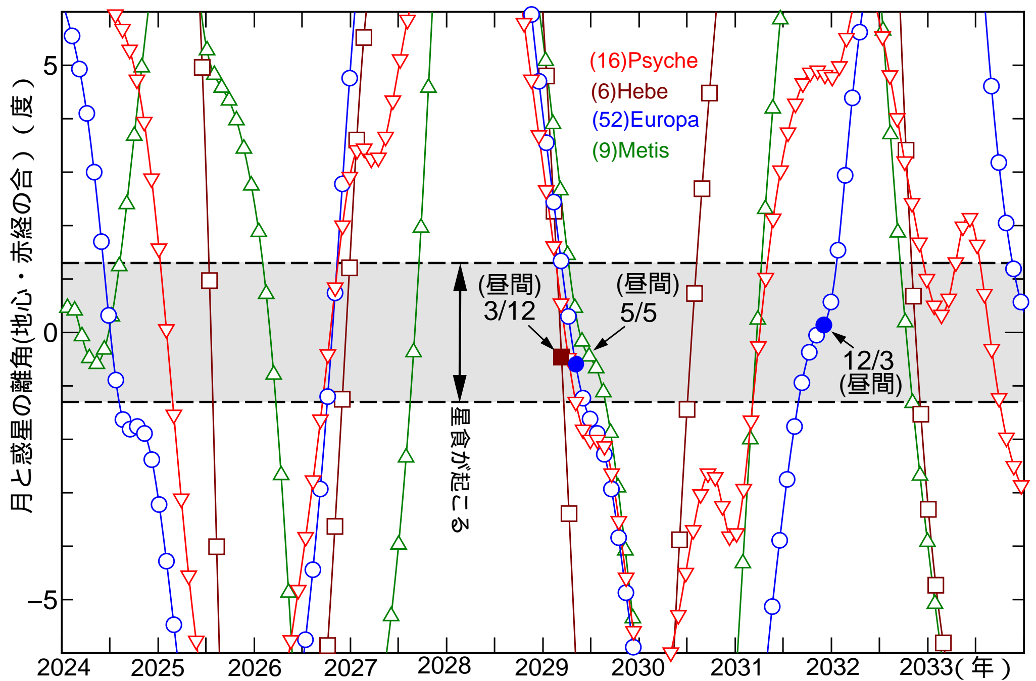
図5 小惑星食ダイアグラム(2) (目盛りは毎年1月1日と7月1日)
