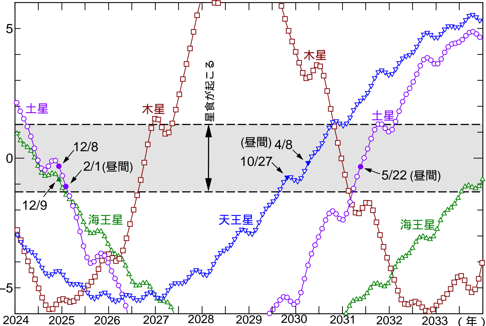
図2 惑星食ダイヤグラム
