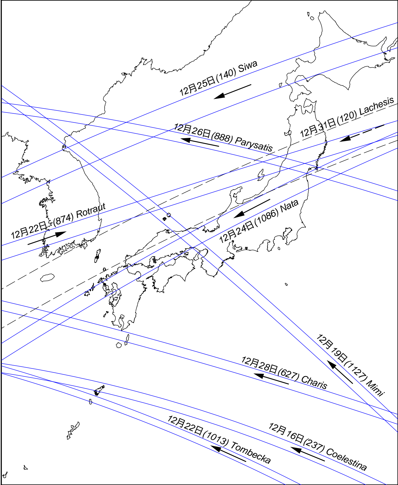
図7 小惑星による主な掩蔽帯経路 ( S.Preston予報ほか ) 2024年12月後半 矢印は影の移動方向を示す
