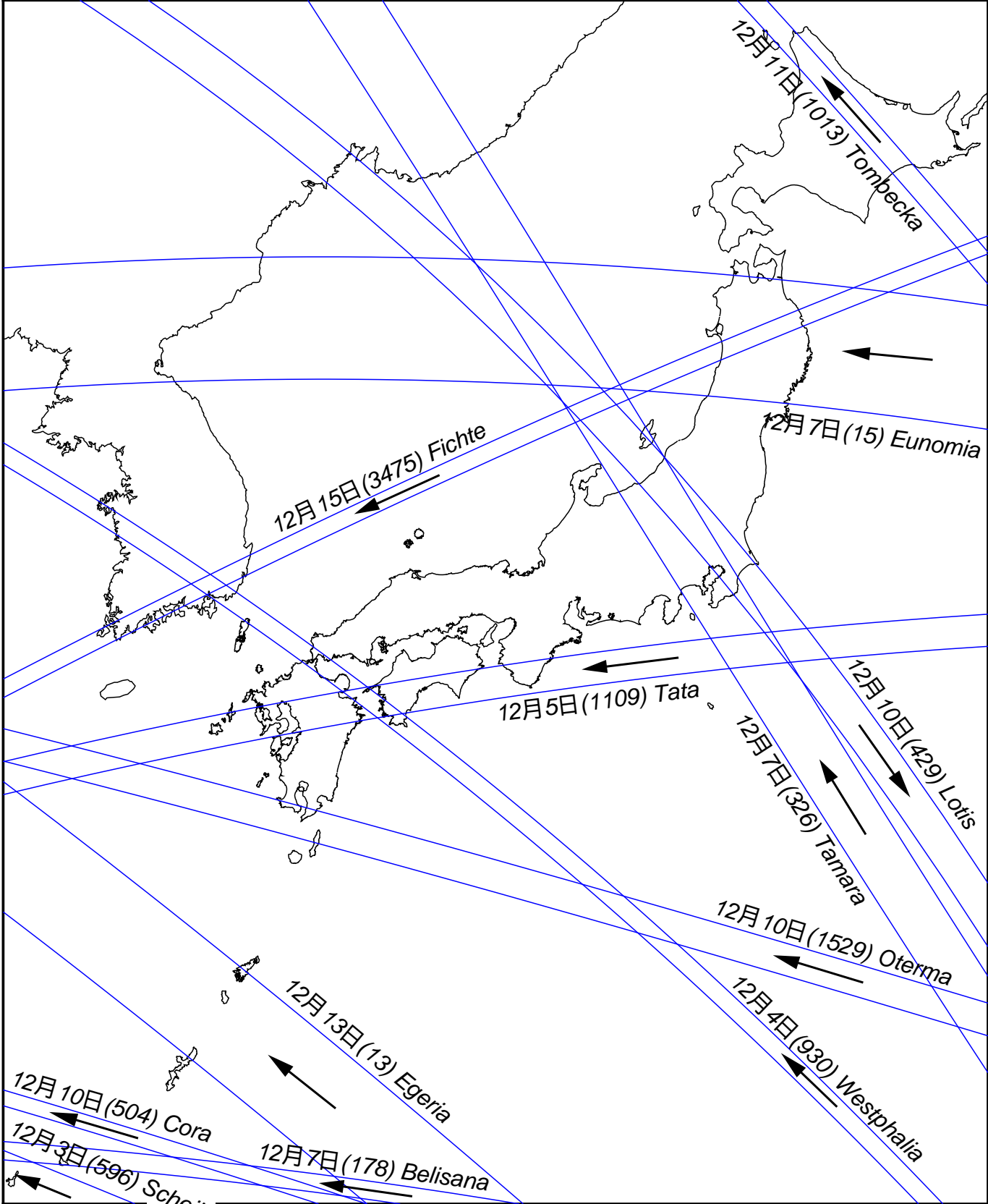
図6 小惑星による主な掩蔽帯経路 ( S.Preston予報ほか ) 2024年12月前半 矢印は影の移動方向を示す
