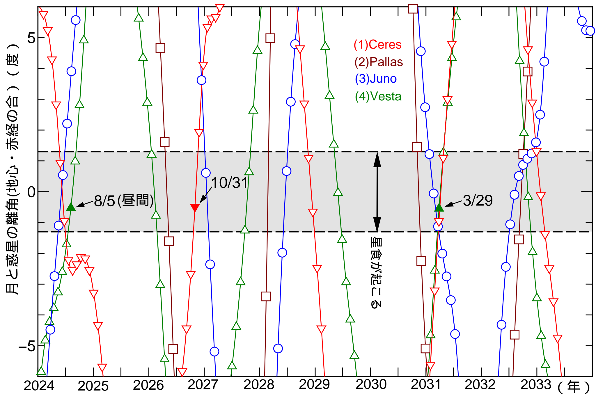
図4 小惑星食ダイアグラム
