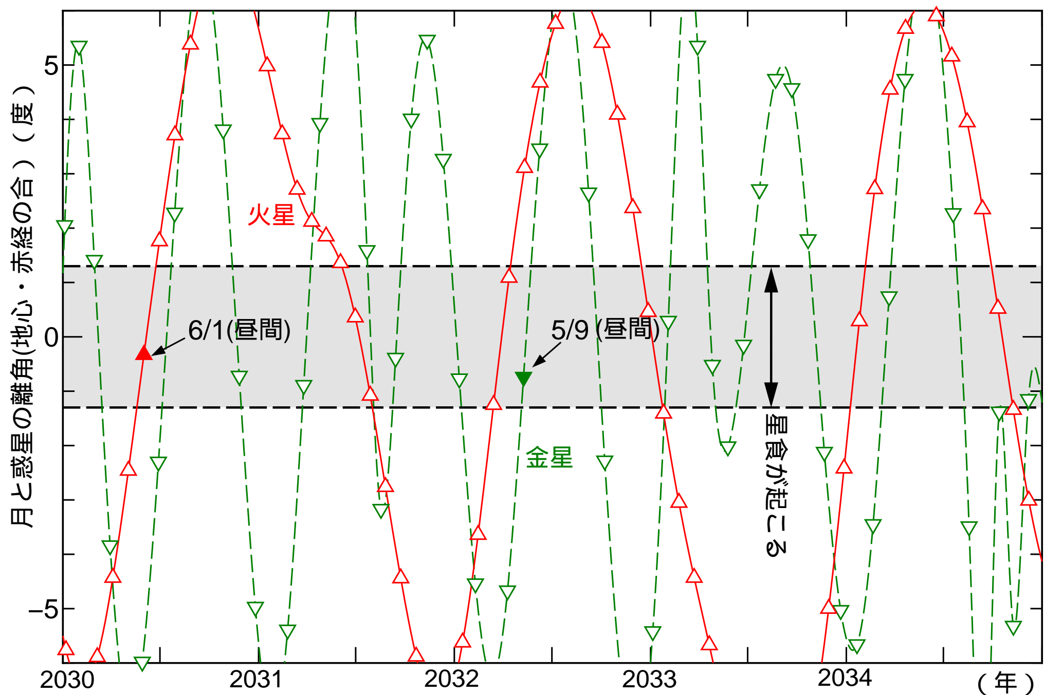
図3b 金星・火星食ダイヤグラム (目盛りは毎年1月1日と7月1日)
