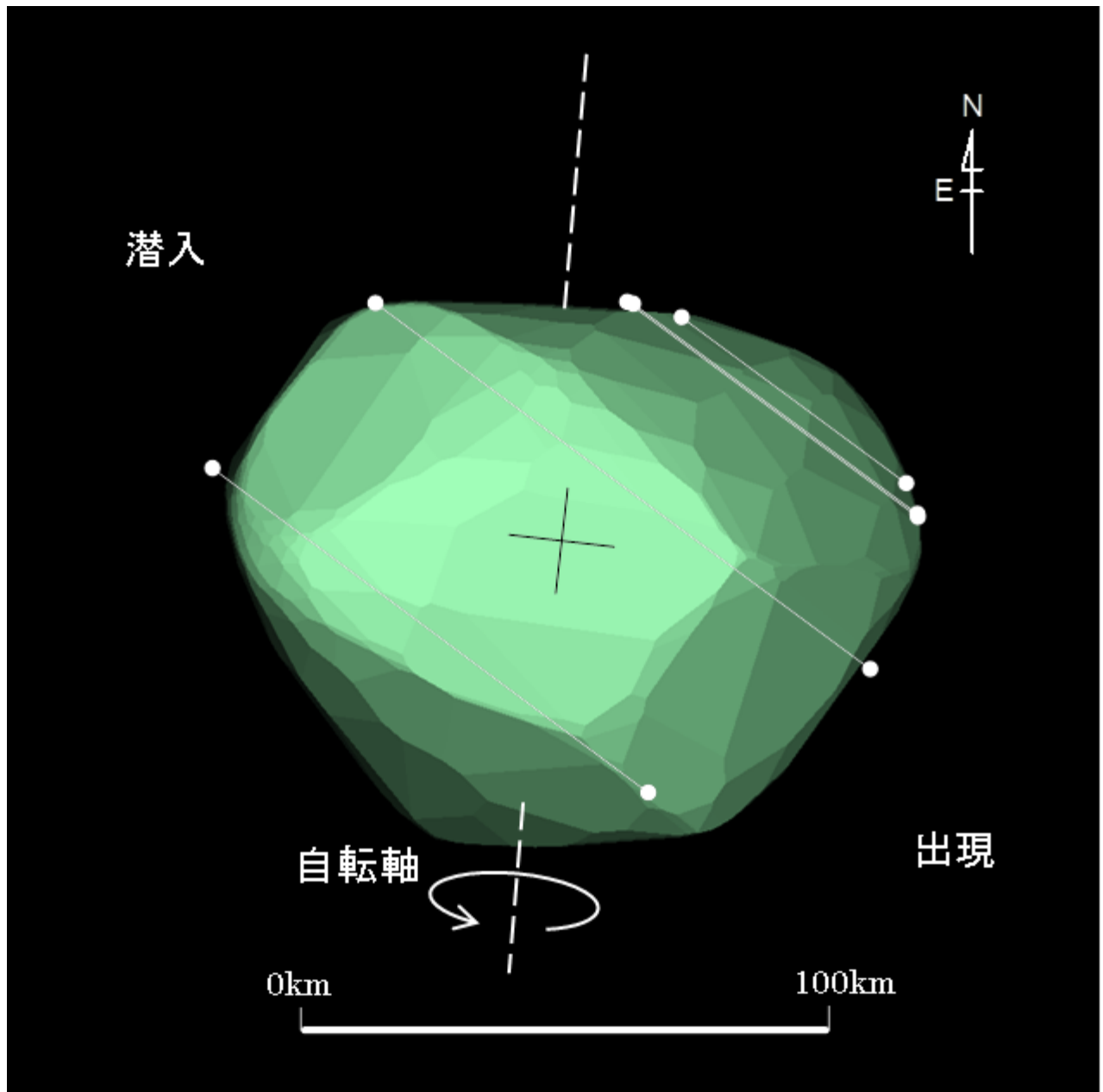
(127)Johanna 2014年9月8日 20h09m12s UT DAMIT Model 445 ( \lambda = 261 、 \beta = -70 ) P = 175.1^\circ 、 \beta_e = 19.3^\circ 、 \lambda_e = -18.7^\circ 、Scale Factor 1:93.2、 k = 0.969 、 B = 76.5^\circ
