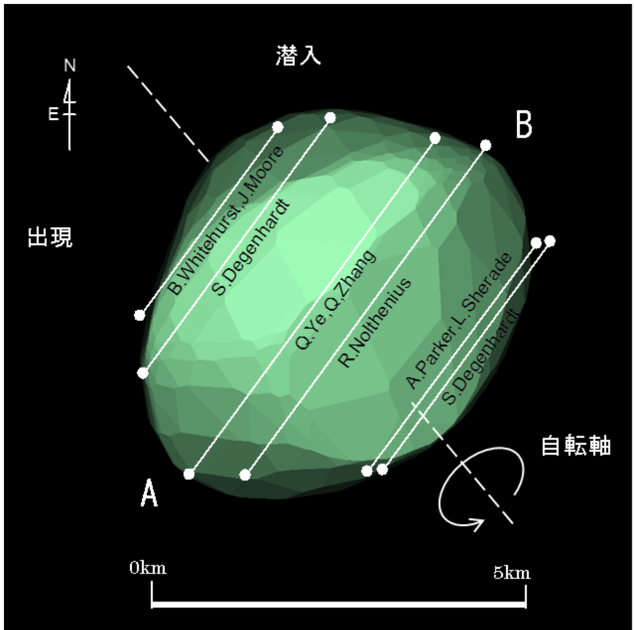
(3200) Phaeton 2019年7月29日 11h20m00s UT DAMIT Model 4394 ( \lambda = 318 , \beta = -47 ) P = 220^\circ , \beta_e = +36^\circ , \lambda_e = -103^\circ , Scale Factor 1: 1.029, k = 0.662 , B = 103.8^\circ
