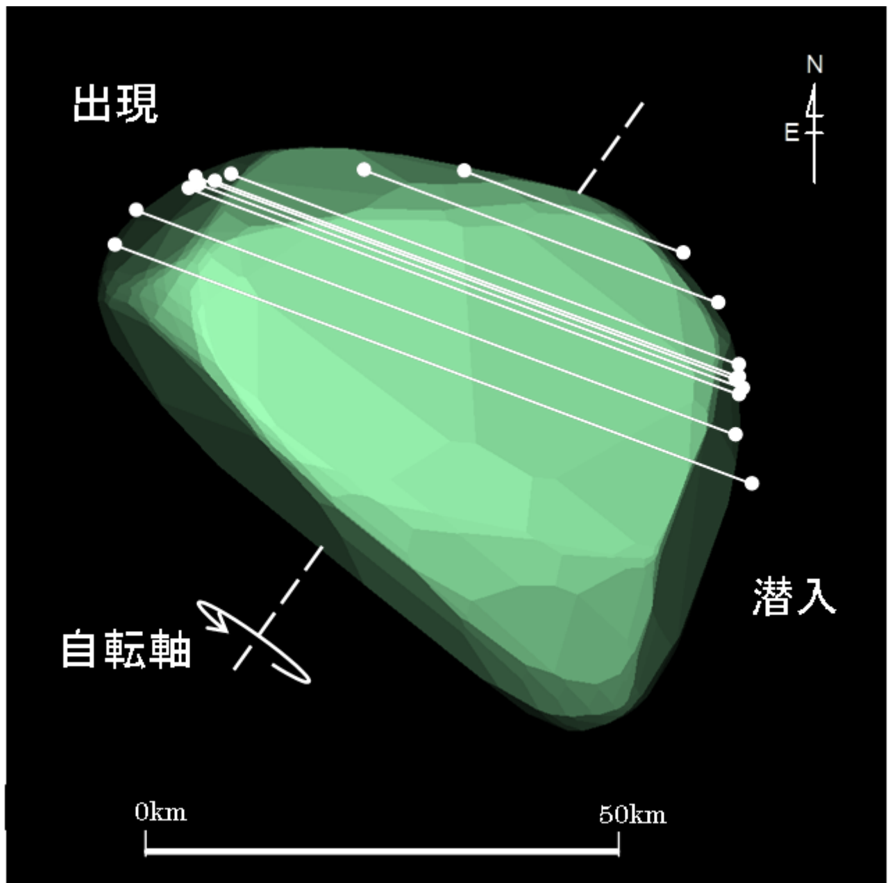
(119)Althaea 2019年11月14日 14h02m20s UT DAMIT Model 324 ( \lambda = 181 、 \beta = -61 ) P = 144^\circ 、 \beta_e = +7^\circ 、 \lambda_e = 338^\circ 、Scale Factor 1: 48.7、 k = 0.937 、 B = 101.9^\circ
