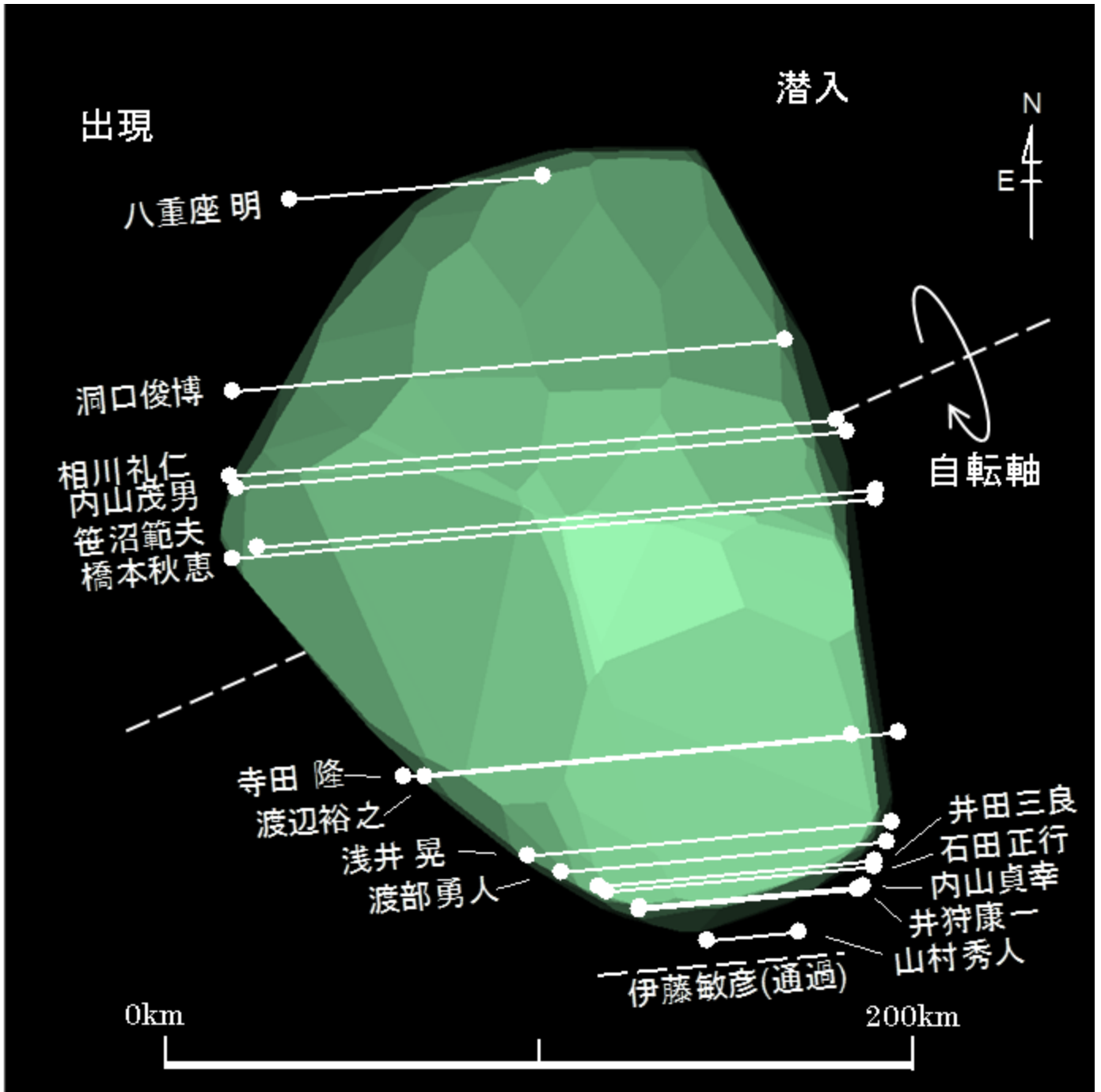
(334) Chicago 2017年12月21日 15h14m28s UT DAMIT Model 4269 ( \lambda = 21 , \beta = +20 ) ※1 P = 294^\circ , \beta_e = -13^\circ , \lambda_e = -158^\circ , Scale Factor 1:143.3, k = 1.000 , B = 123.52^\circ
