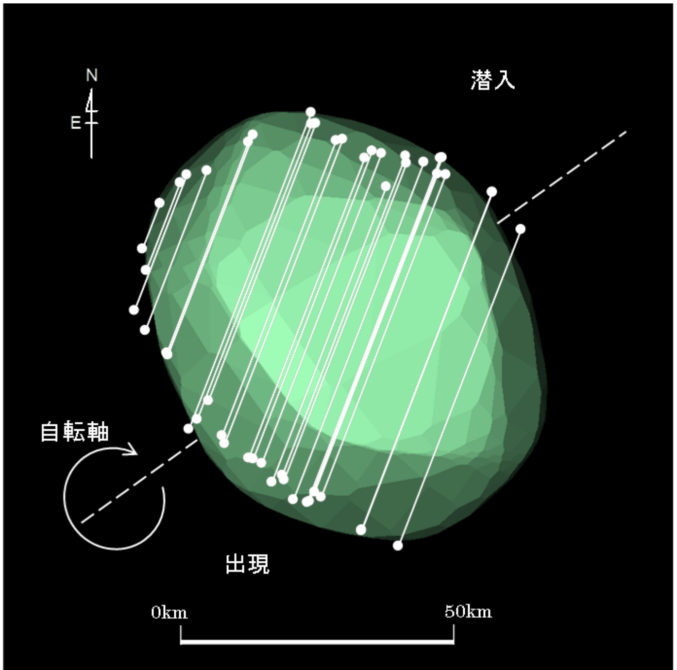
(498) Tokio 2004年2月17日 16h35m27s UT DAMIT Model 6123 ( \lambda = 275 、 \beta = -10 ) P = 125.2^\circ 、 \beta_e = -11.5^\circ 、 \lambda_e = -261.6^\circ 、Scale Factor 1: 58.2、 k = 0.985 、 B = 102.3^\circ
