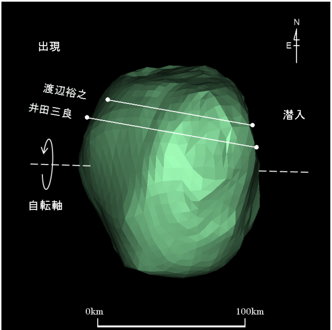
(22) Kalliope 2021年9月9日 18h46m34s UT VLT/SPHERE Model ( \lambda = 195.0606 、 \beta = +3.3321 ) P = 88.0^\circ 、 \beta_e = +11.1^\circ 、 \lambda_e = -265.4^\circ 、Scale Factor 1: 1.0、 k = 0.965 、 B = 92.1^\circ
