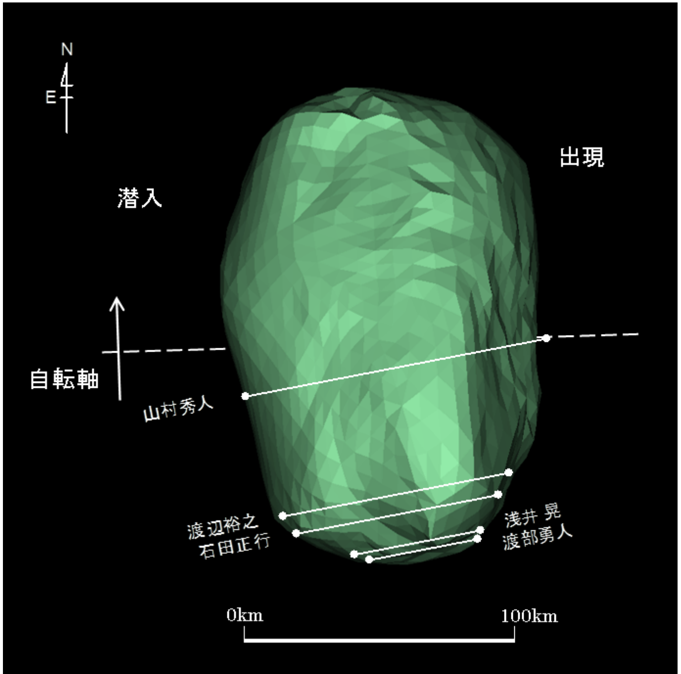
(22) Kalliope 2022年4月22日 10h53m16s UT VLT/SPHERE Model ( \lambda = 195.0606 、 \beta = +3.3321 ) P = 92.9^\circ 、 \beta_e = +0.8^\circ 、 \lambda_e = -308.7^\circ 、Scale Factor 1: 1.0、 k = 0.969 、 B = 272.8^\circ
